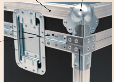
Eckverbindung 6fach genietet
